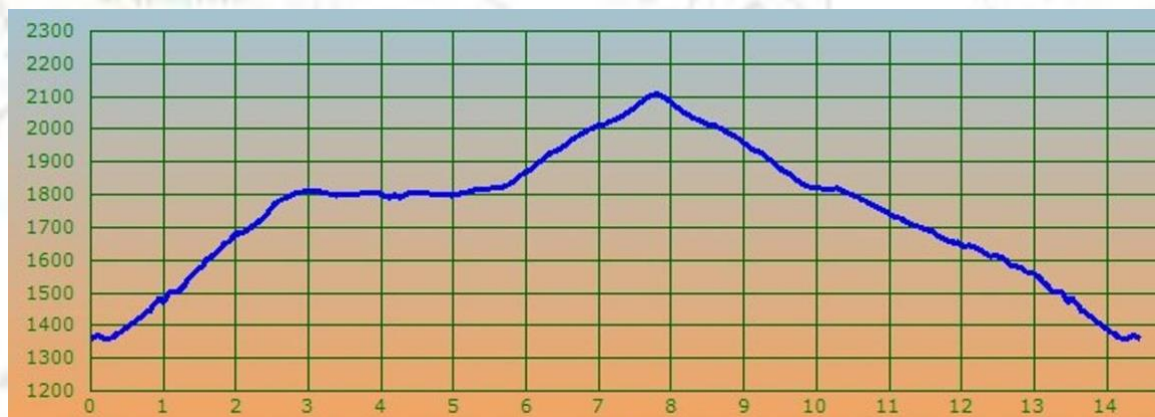
Profilo altimetrico
